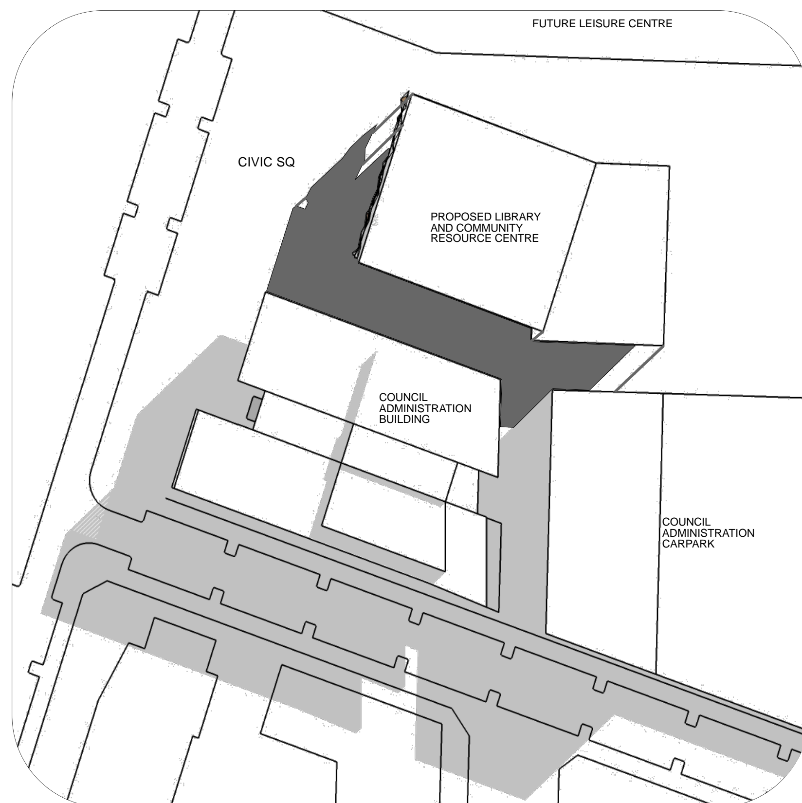
Winter Solstice 9am
